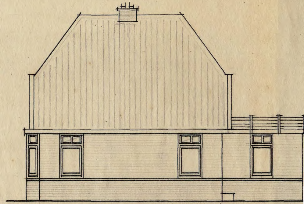
ZUGEVEL -
