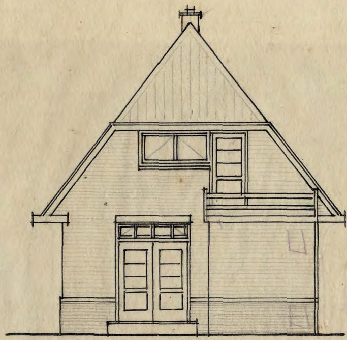
ACHTERGEVEL -
