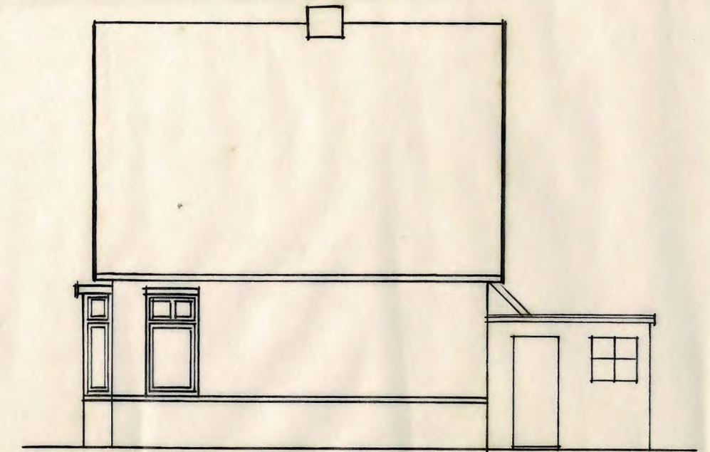
ZYGEVEL
